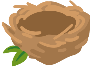
nest
